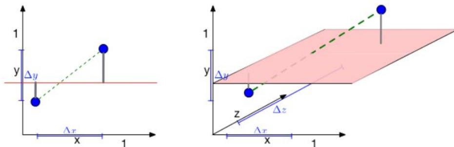
Figura 3-17: Efeito do aumento de dimensão nas distâncias de um espaço.
